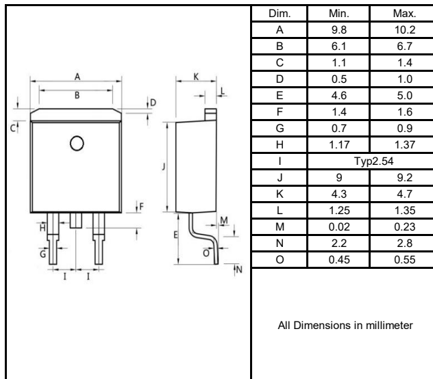
T0-263C
