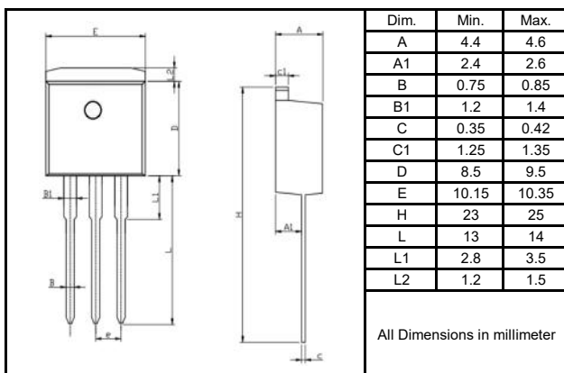
T0-262C
